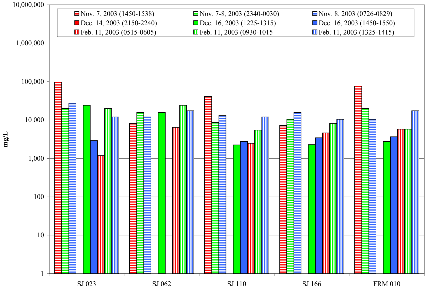
Figure D-2. E. coli
